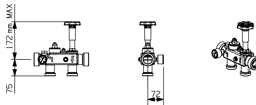
Module SIMPLY CONNECT 2" Vues échelle 1/10 eme
