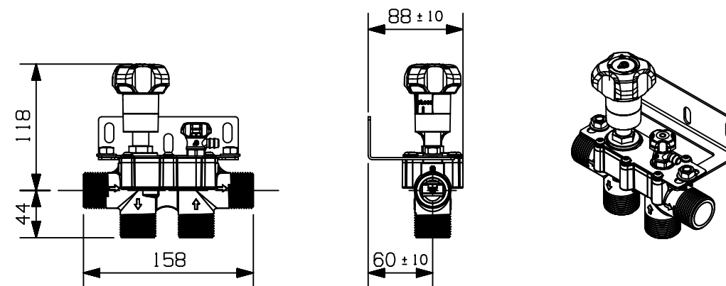
Module By-pass 1" Ech:1/5
