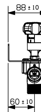
MODULE BY-PASS 1" ECH 1/5
